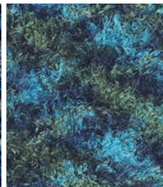
ocean color 00180
